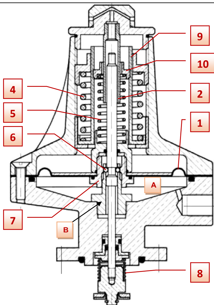
Конструкция пилота ПЗК типа BLC
