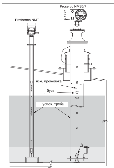
Резервуар с фиксированной крышей
