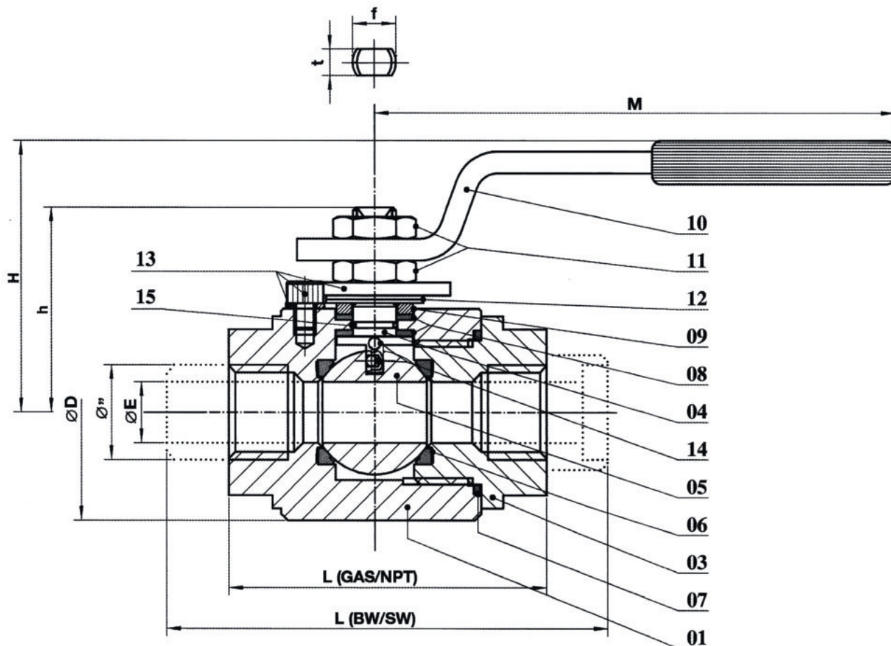
DIMENSIONI - DIMENSIONS - DIMENSIONS - ABMESSUNGEN
