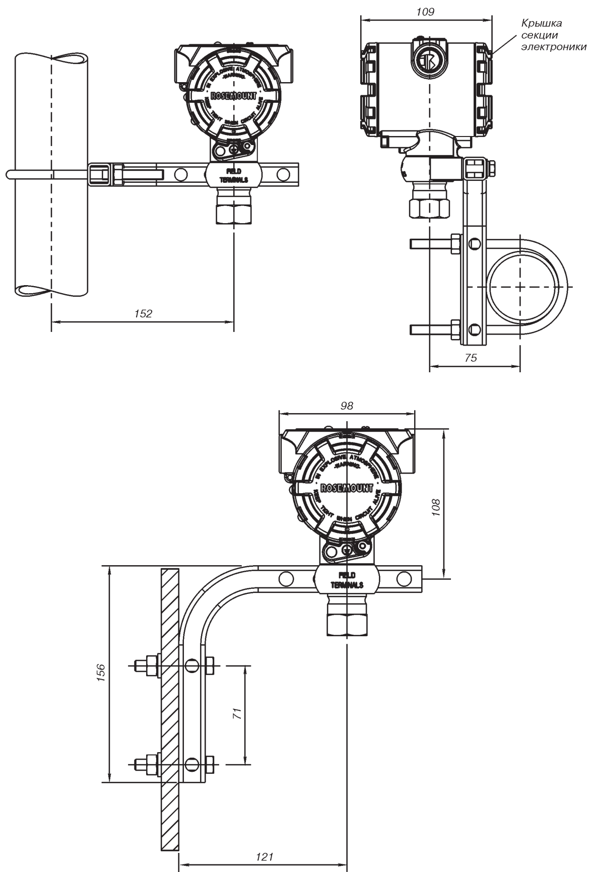
Рис.8. Монтаж преобразователя 2051G на двухдюймовой трубе и панели (код опции В4).
