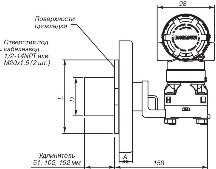
Рис.10. Преобразователь давления модели 2051L с удлинителем.
