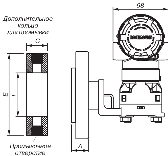
Рис.9. Преобразователь давления модели 2051L с фланцем заподлицо.
