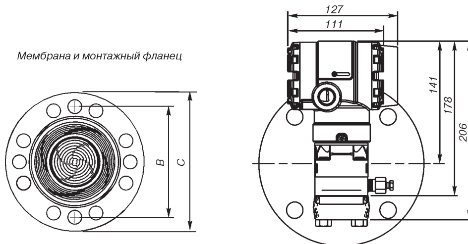
Рис.11. Преобразователь давления модели 2051L для измерения уровня.
