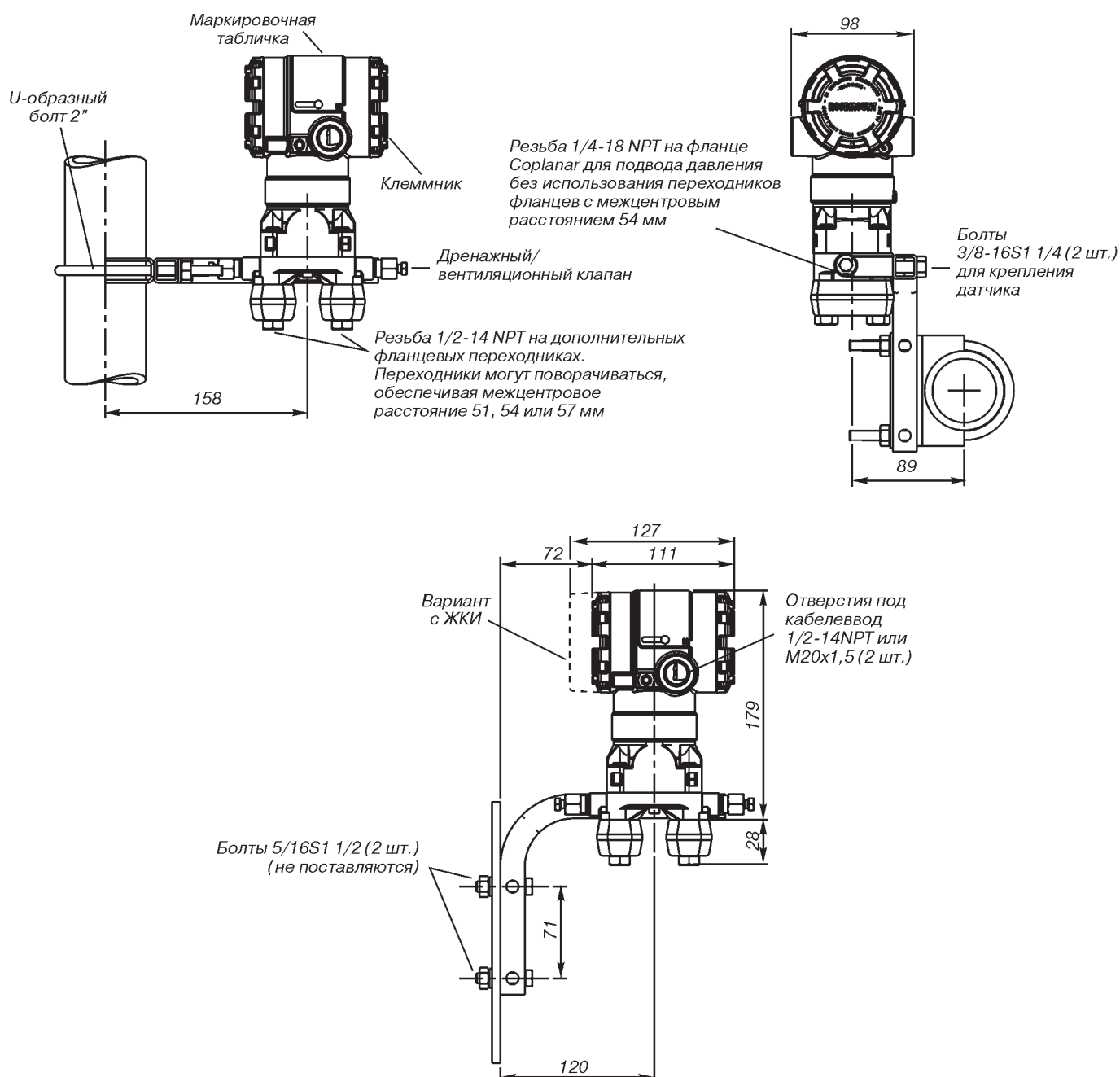
Рис.5. Преобразователь давления модели 2051C с фланцем Corlana с дополнительным кронштейном (B4) для монтажа на 2-дюймовой трубе или панели.
