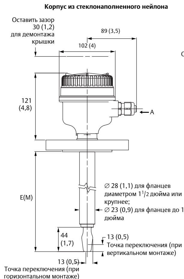
Рис. А-10. Фланцевый монтаж (увеличенная длина)
