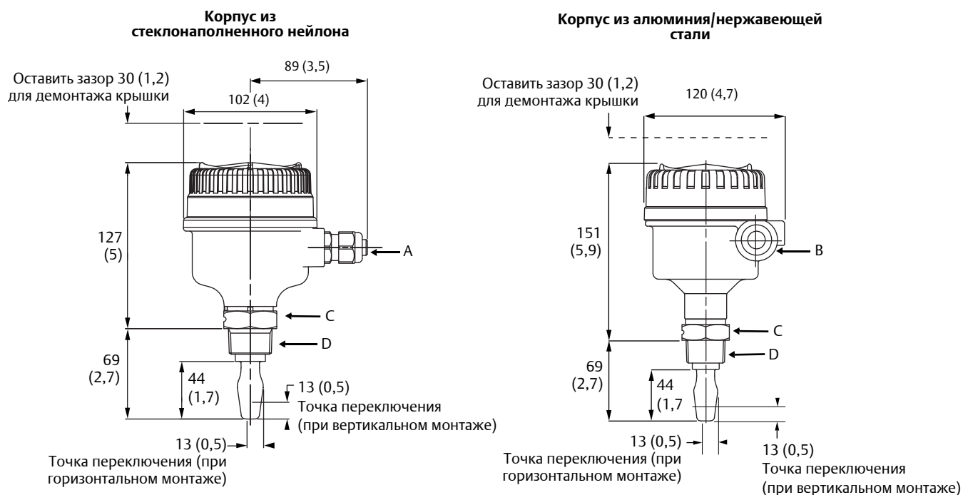
Рис. А-3. \frac{3}{4} - и 1-дюйм. Резьбовой монтаж (стандартная длина)
