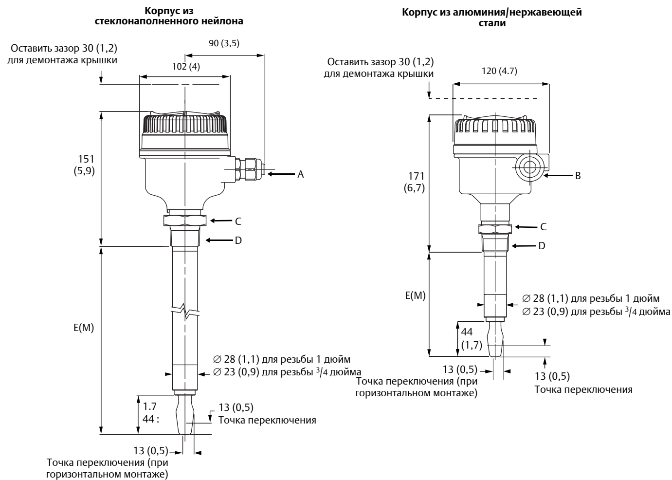
Рис. А-4. \frac{3}{4} - и 1-дюйм. Монтаж на резьбовом соединении (увеличенная длина)
