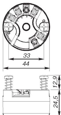
Соединительная головка (код опции А)
