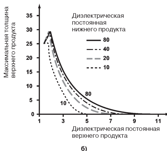
Рис.9. Максимальная толщина верхнего продукта для одинарного гибкого (а) и для двойного гибкого (б) зонда в м.
