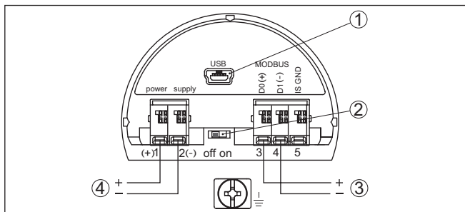
Рис. 8: Отсек подключения
