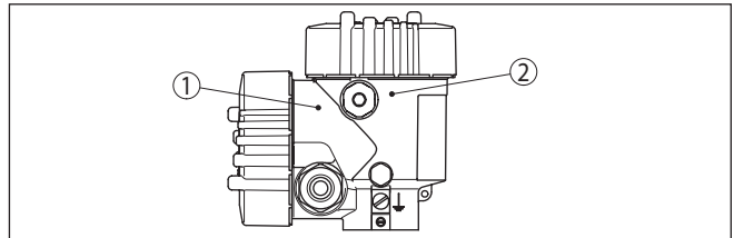
Рис. 6: Позиция отсека подключения (электроника Modbus) и отсека электроники (электроника датчика)
