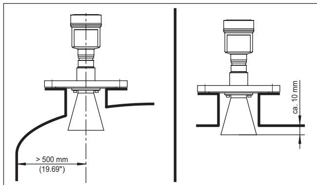
Рис. 2: Расстояние от антенны до стенки емкости/крыши емкости
